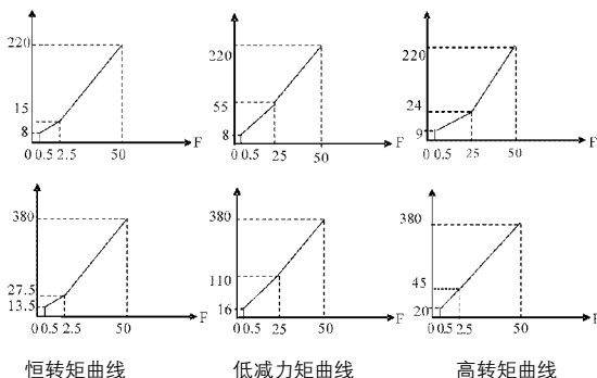
恒转矩曲线
